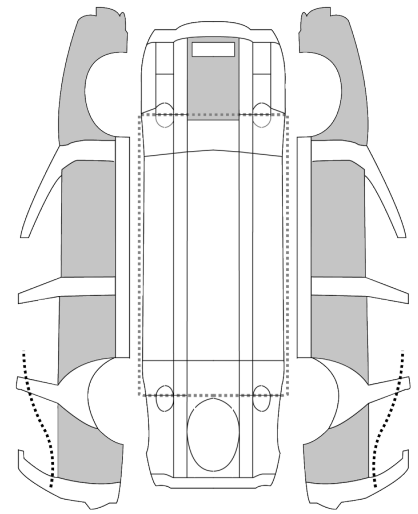
車骨結構圖
