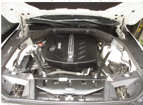
引擎室
