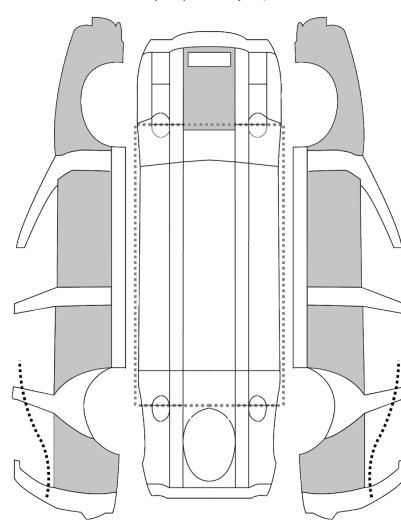
車骨結構圖
